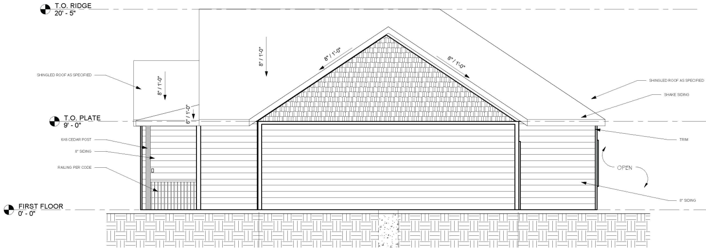
RIGHT ELEVATION
